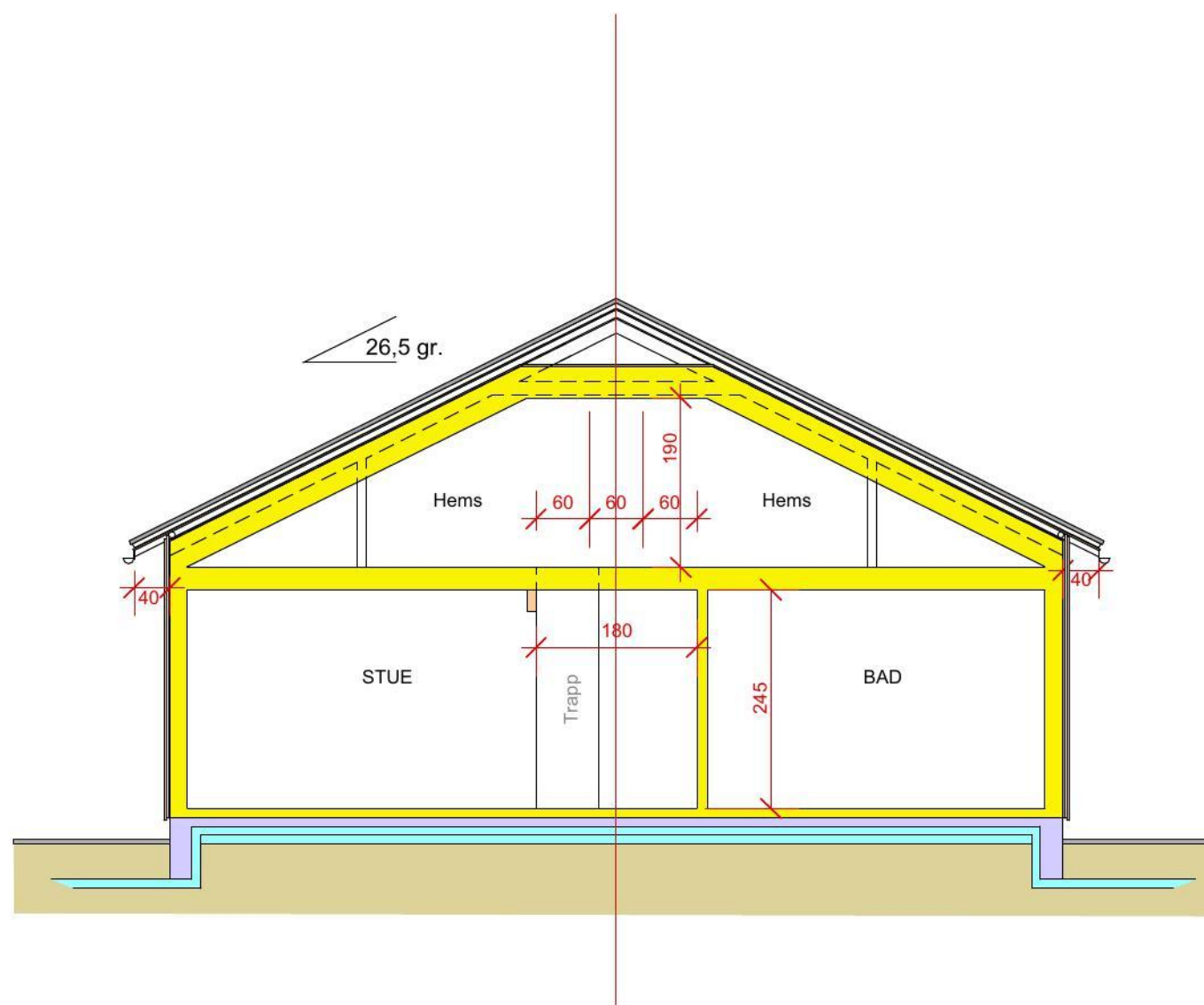
SNITT A-A (Sett fra siden mot vannet)
